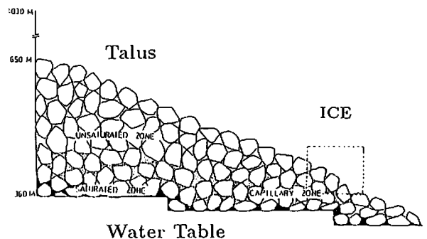
第2図 崖錐の想像断面図。縦軸は海拔高度。岩屑の隙間は雨や地下水による水分の供給で湿っており、そこを空気は自由に通り抜けることができる。30°Cを越える外気温と、約8°Cの地下水に挟まれた破線領域で氷が成長する。
