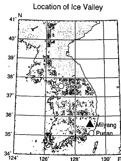
第1図 Ice Valley がある韓国密陽郡 (Milyang) の位置。
