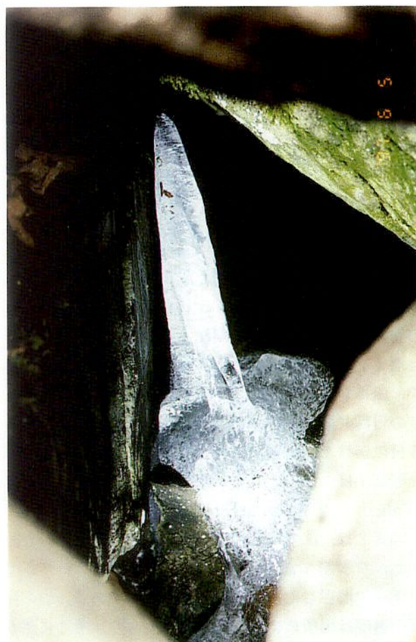
写真2 風穴内部で下から伸びた約20 cm の氷筈。光が届く深さなので、岩には緑の苔が生えている。他につらら状のものや、残雪のように白くなった氷もある。
