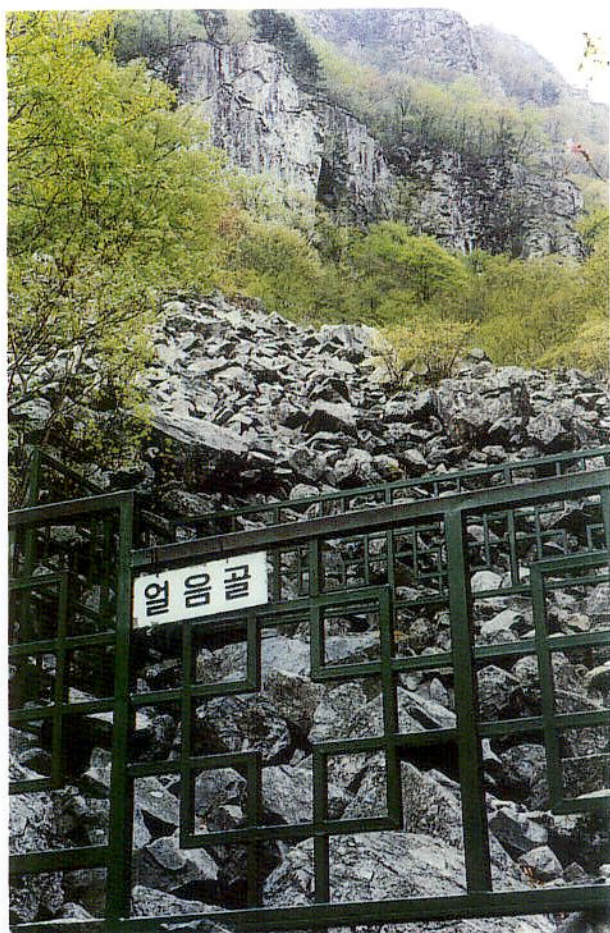
写真1 海拔高度410 m 地点の崖錐の様子。直径1 m 程の岩屑が重なり合っており、この岩の隙間で水が発達する。水が最も発達する一角では、観光客が立ち入らぬように柵がしてある。
