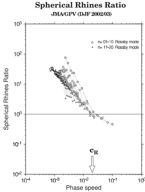
図 2: 球面 Rhines 比と球面 Rhines スケール
