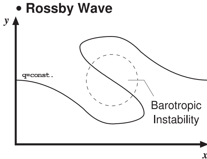
図 4: Rossby 波の碎波条件
