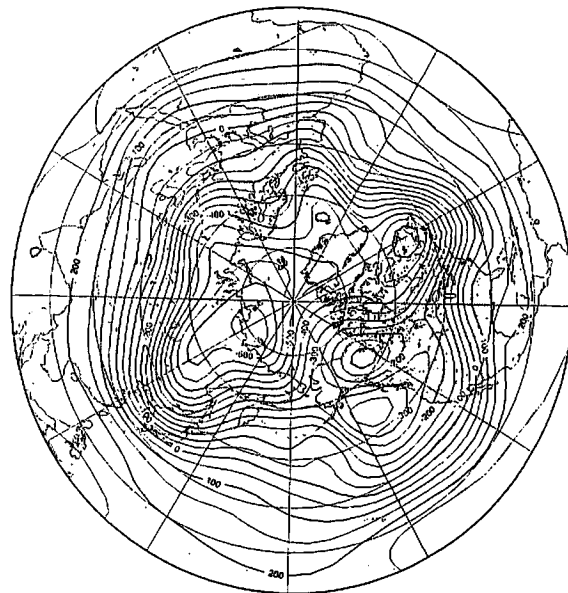
図-1. 順圧 B-モデルに現れたダイポール型のブロッキング (Tanaka 1998)。
